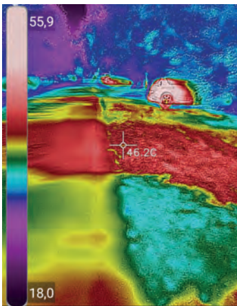
Aufnahme einer Wärmebildkamera eines Parkplatzes mit Asphalt in der Mitte und Schotterrasen am Rand. Dort wo asphaltiert ist und kein Schatten hinfällt ist es am heißesten.
